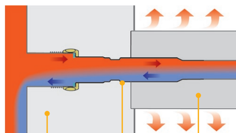
Solarspeicher mit Isolierung Kombifitting Anschlussrohr mit Isolierung
