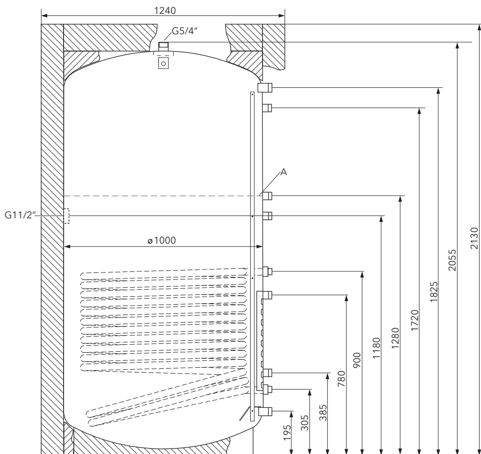
Abb. 8 RATIO 1500 (ohne Wärmeübertrager) bzw. 1500-G im Längsschnitt mit Maßen [mm]; = Bezugsebene in Tab. 1 für Nachheizvolumen.
