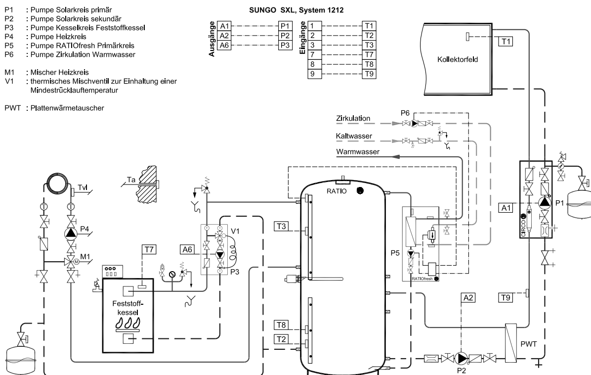
Abb. 12 Systemlösung mit RATIO Pufferspeicher, Frischwasserstation RATIOfresh 250/400, Feststoffkessel, einem gemischten Heizkreis und einer größeren Kollektorfläche. Die Warmwasserbereitung erfolgt im Durchflussprinzip. Solarenergie wird über einen leistungsstarken Plattenwärmeübertrager an den Pufferspeicher übergeben. Der Feststoffkessel nutzt das gesamte Speichervolumen. Über einen eingebauten Elektroheizstab kann bei längeren Abwesenheitszeiten ein Heizbetrieb gewährleistet werden.
