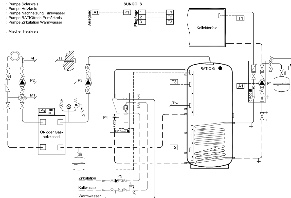
Abb. 9 Solaranlage für die Warmwasserbereitung im hygienischen Durchflussverfahren. Systemlösung mit RATIO Pufferspeicher, Frischwasserstation RATIOfresh 250/400 und einem Öl- oder Gasheizkessel. Der Regler der Frischwasserstation sorgt für konstante Warmwasser-Zapftemperaturen und die Ansteuerung der Zirkulationspumpe. Die Leistungsregelung der Frischwasserstation sorgt zudem für niedrige Rücklauftemperaturen in den Pufferspeicher und erhöht damit den solaren Anlagenenertrag.
