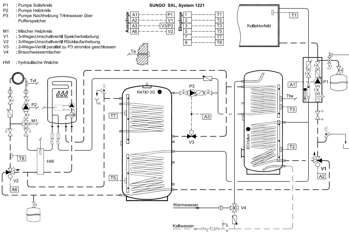
Abb. 11 Solaranlage für die Warmwasserbereitung und Heizungsunterstützung: 2-Speicher-System mit ECOplus-Solarspeicher, RATIO Pufferspeicher, Gastherme und einem gemischten Heizkreis. Die Solarenergie wird vom Solarregler SUNGO SXL optimal auf beide Speicher verteilt und über eine Anhebung der Heizungs-Rücklauftemperatur für den Heizkreis genutzt. Solarwärme aus dem Puffer steht zusätzlich auch für die Warmwasserbereitung zur Verfügung.
