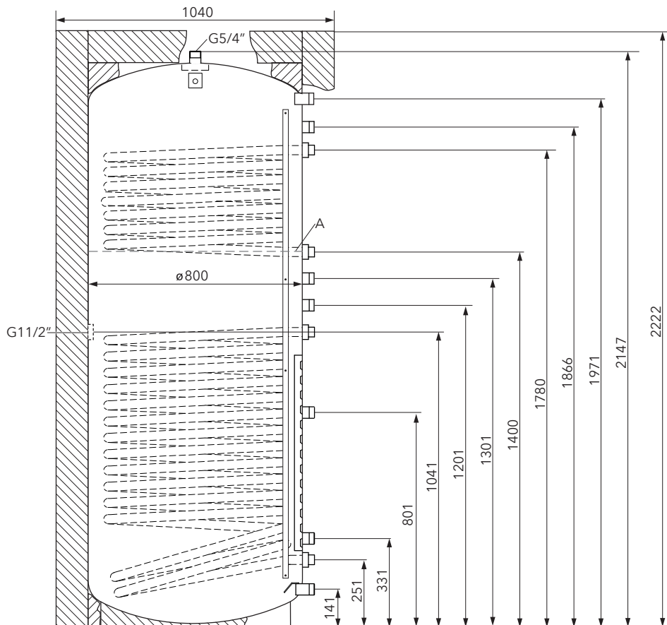
Abb. 7 RATIO 1000 (ohne Wärmeübertrager) bzw. 1000-2G im Längsschnitt mit Maßen [mm]; A = Bezugsebene in Tab. 1 für Nachheizvolumen.
