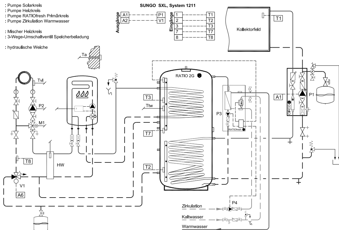
Abb. 10 Solaranlage für die Warmwasserbereitung und Heizungsunterstützung. Systemlösung mit RATIO Pufferspeicher und Frischwasserstation RATIOfresh 250/400 in Verbindung mit einer Gastherme und einem gemischten Heizkreis. Die Warmwasserbereitung erfolgt im hygienischen Durchflussverfahren. Solarenergie wird über eine Rücklaufanhebung des Heizkreises genutzt.
