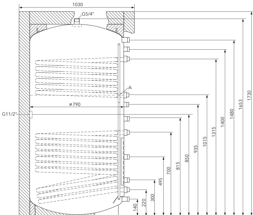
Abb. 6 RATIO 700 (ohne Wärmeübertrager) bzw. 700-2G im Längsschnitt mit Maßen [mm]; A = Bezugsebene in Tab. 1 für Nachheizvolumen.
