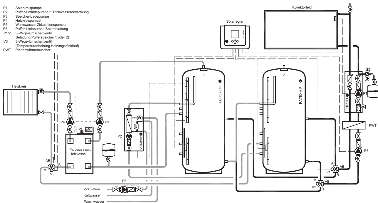
Bild 10 Solaranlage für Warmwasserbereitung und Heizungsunterstützung. System mit Öl- oder Gaskessel, 2 Pufferspeicher RATIO HP und Frischwasserstation RATIOfresh. Der Pufferspeicher 1 wird vom Kollektorfeld vorrangig beladen. Die Warmwasserbereitung erfolgt im elektronisch geregelten Durchflussverfahren. Der Regler der Frischwasserstation sorgt nicht nur für eine energetisch günstige Entladung der Pufferspeicher bei einer Warmwasserzapfung, er betreibt auch die Warmwasser-Zirkulationspumpe drehzahl geregelt. Bei ausreichenden Temperaturen im Vorrang-Pufferspeicher wird Solarwärme für die Heizung über eine Anhebung der Heizungs-Rücklauftemperatur eingebracht.
