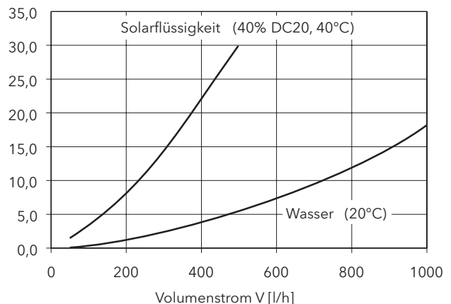
Bild 6 Druckverlust der CONVECTROL III-Konvektionsbremse bei Durchströmung mit Wasser und mit Solarflüssigkeit
