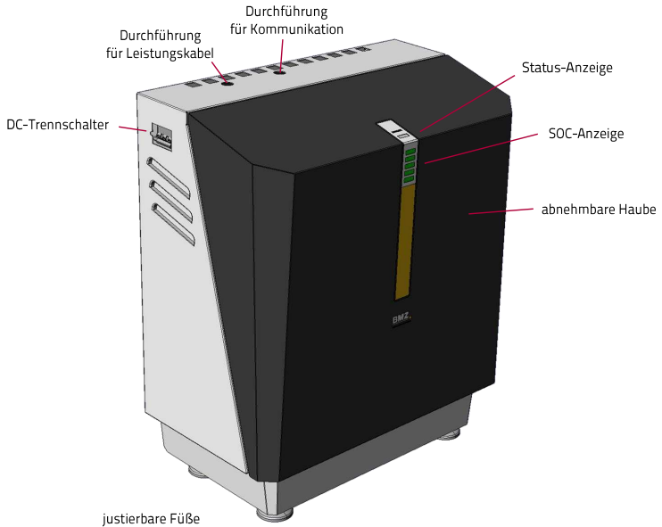
Abbildung 1: Gesamtansicht Batteriesystem
