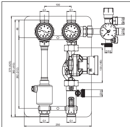
Fig. 4.3 Station solaire avec purgeur d'air, 130 (180) mm DN 25
